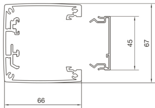
DAS452700ELN
