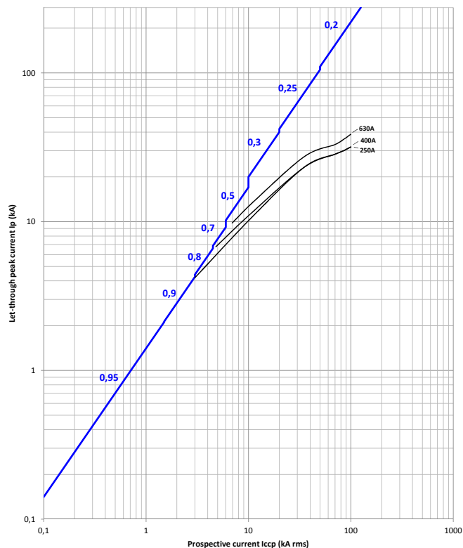
x630 LSnl
