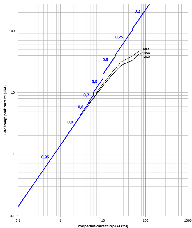
x630 LSnl
